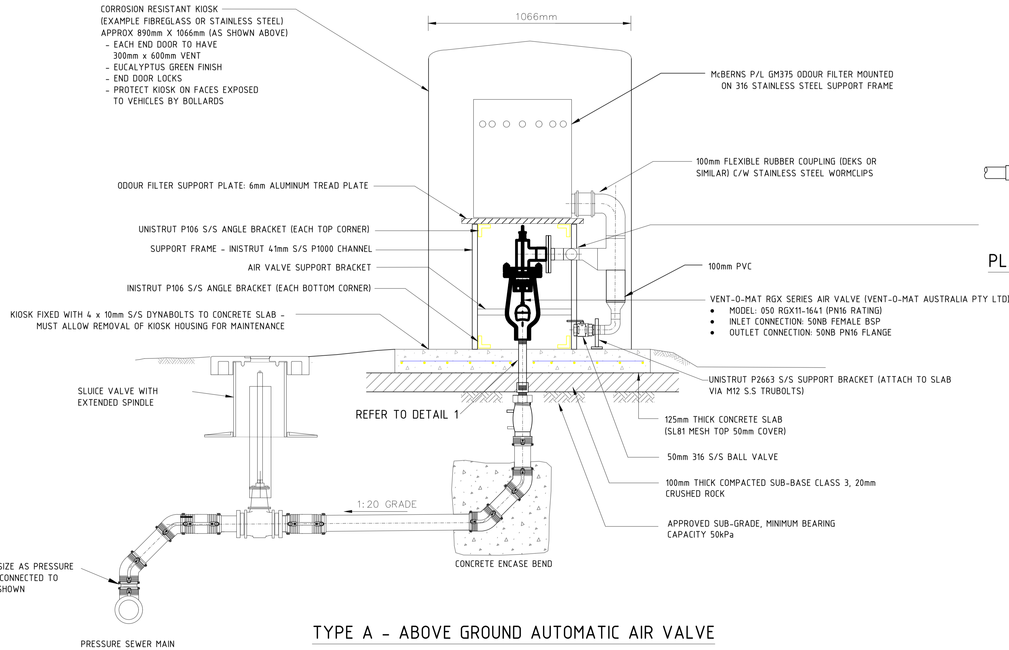
FIBREGLASS KIOSK
