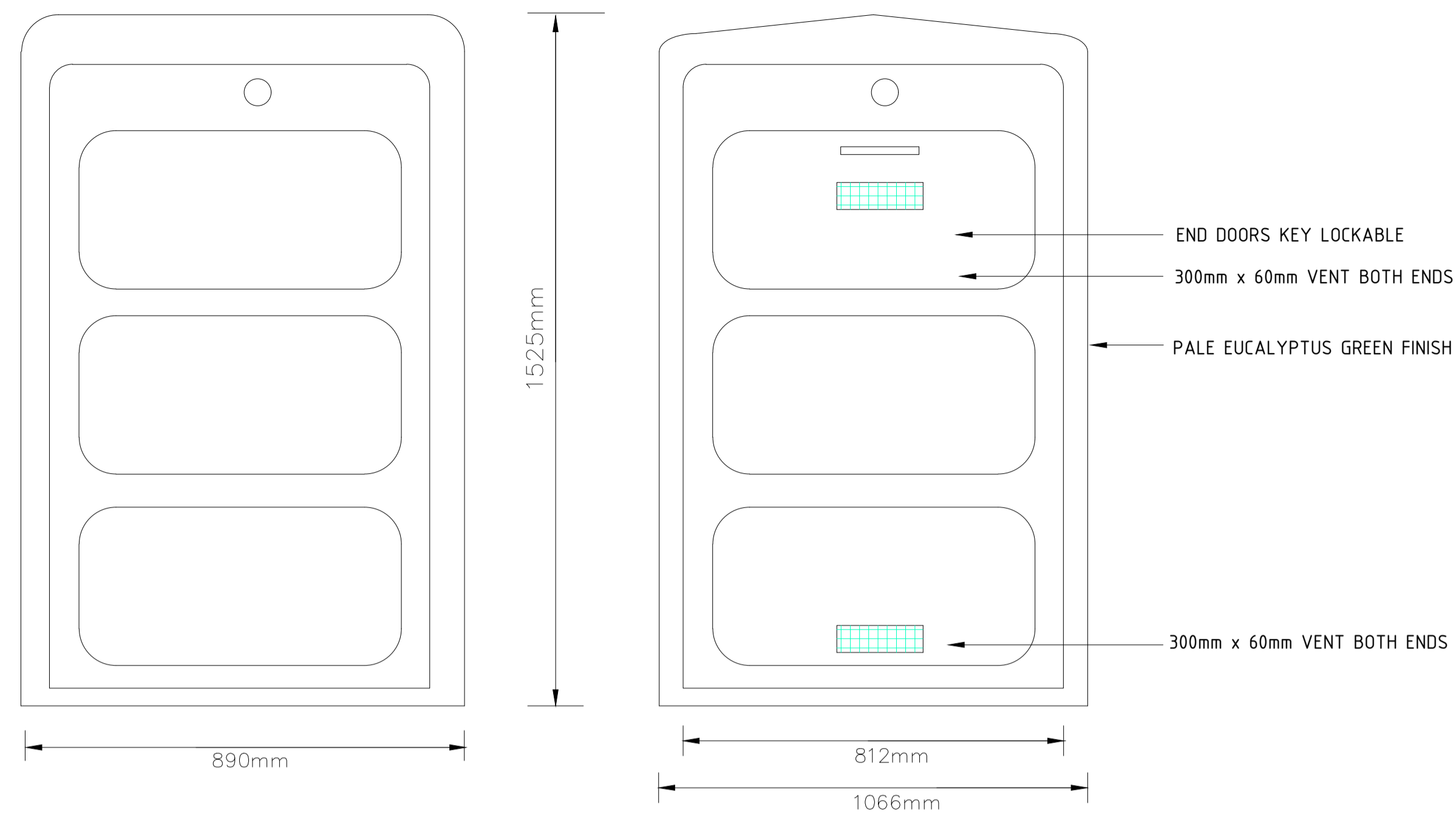
FIBREGLASS KIOSK
